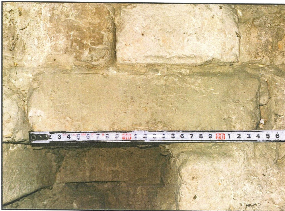
Fot. nr 15 Odkrywka muru ceglano. Wymiary cegły 24 cm x 7 cm.
