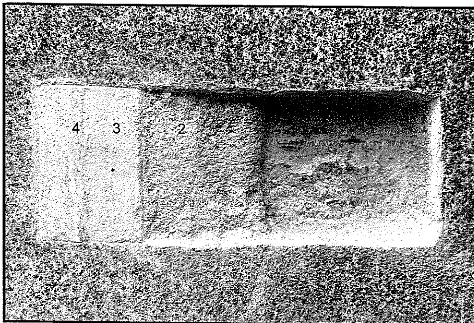
Fot.nr 1 Odkrywka sondażowa tynku elewacji frontowej (zachodniej).
