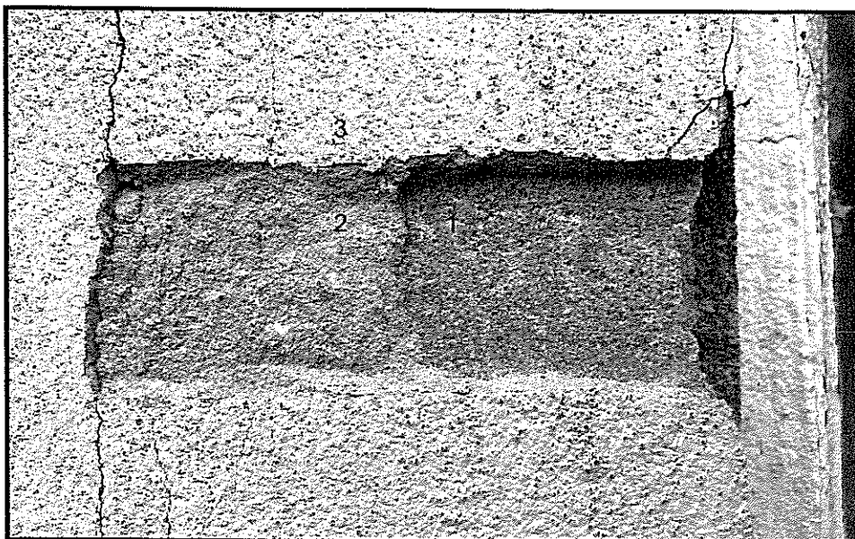
Fot. nr 10 Odkrywka sondażowa detalu architektonicznego (belkowania okna) elewacji północnej.
