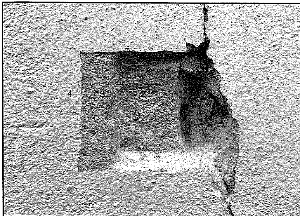
Fot.nr 11 Odkrywka sondażowa elewacji południowej.
