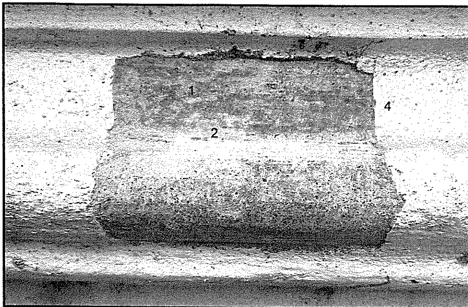
Fot.nr 9 Odkrywka sondażowa detalu architektonicznego (belkowania okna) elewacji północnej.
